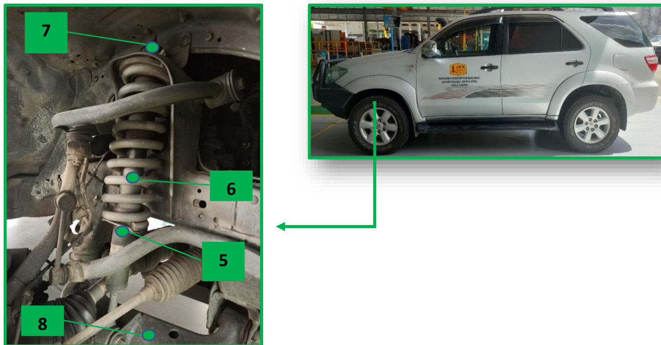
Gambarajah 12 : Komponen Bagi Sistem Suspension Toyota Fortuner (2)
