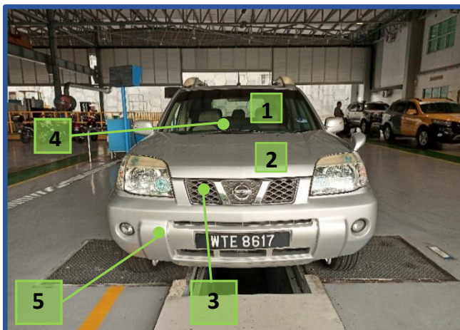
Gambarajah 42 : Komponen Bagi Sistem Badan Kenderaan Nissan Xtrail (1)
