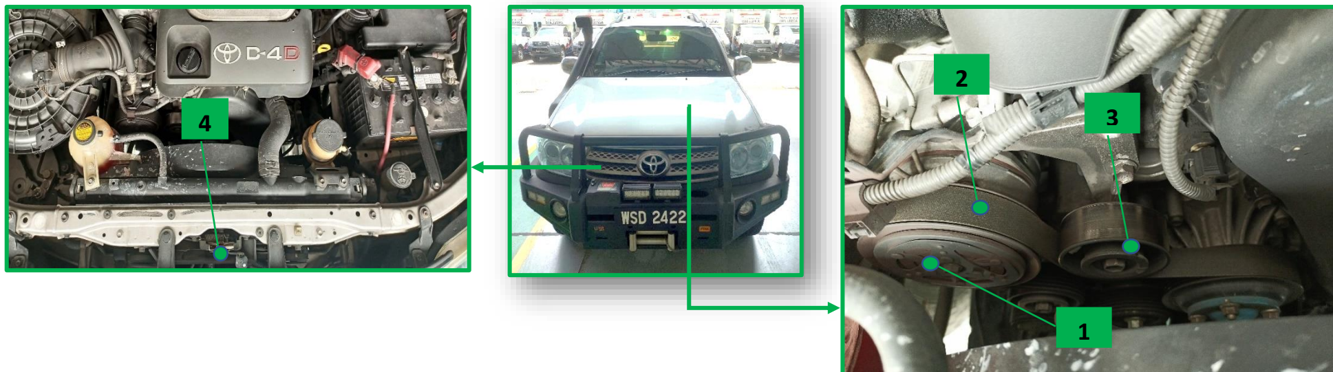
Gambarajah 7 : Komponen Bagi Sistem Penyaman Udara Toyota Fortuner (1)
