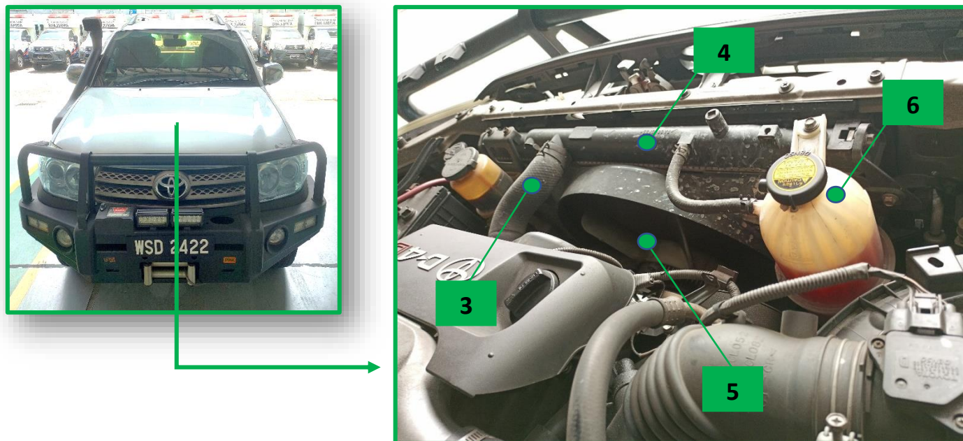
Gambarajah 14 : Komponen Bagi Sistem Penyejukan Enjin Toyota Fortuner (2)
