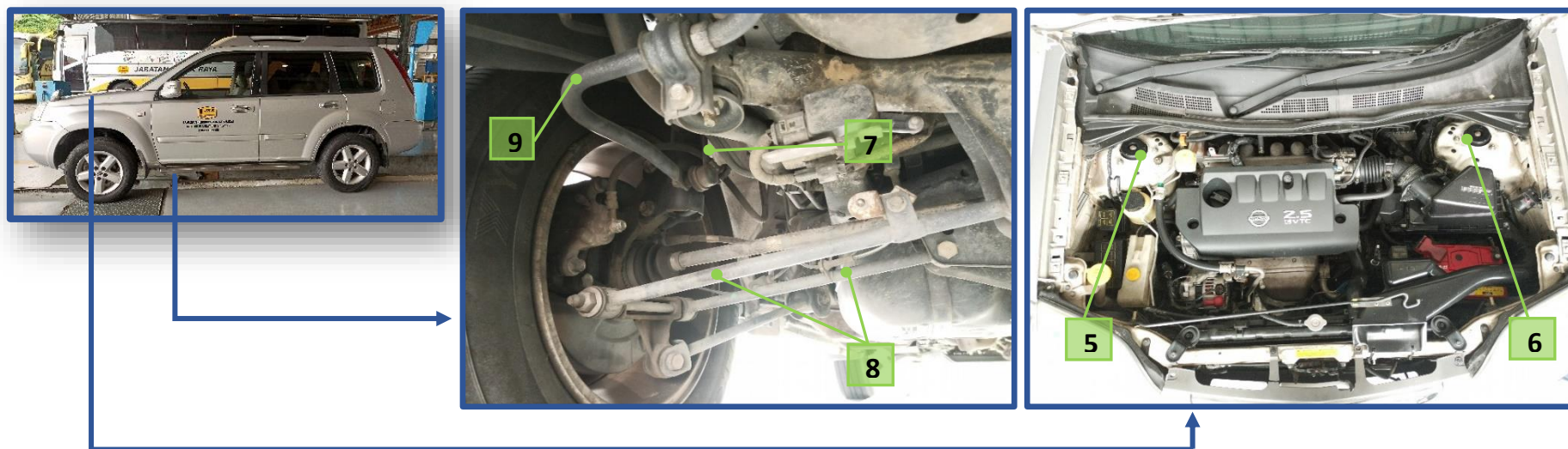
Gambarajah 34 : Komponen Bagi Sistem Suspension Nissan X-trail (2)
