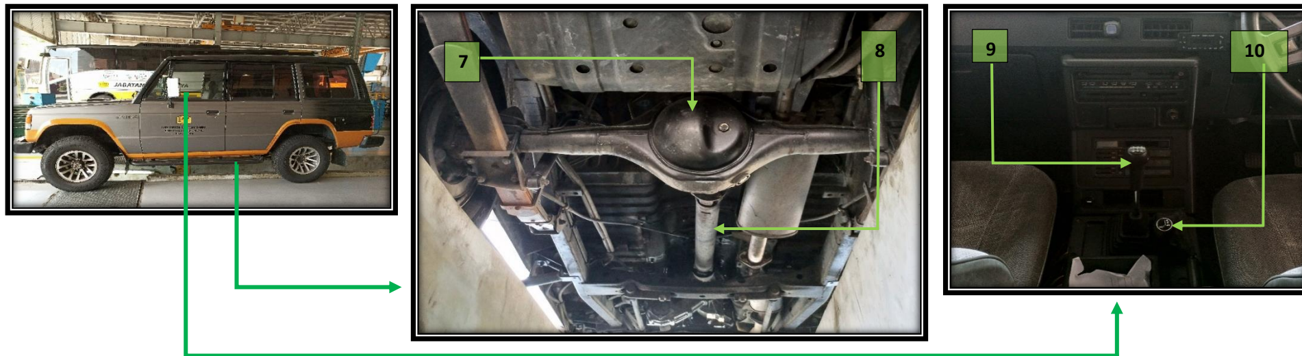
Gambarajah 48 : Komponen Bagi Sistem Tranmisi Mitsubishi Pajero (2)
