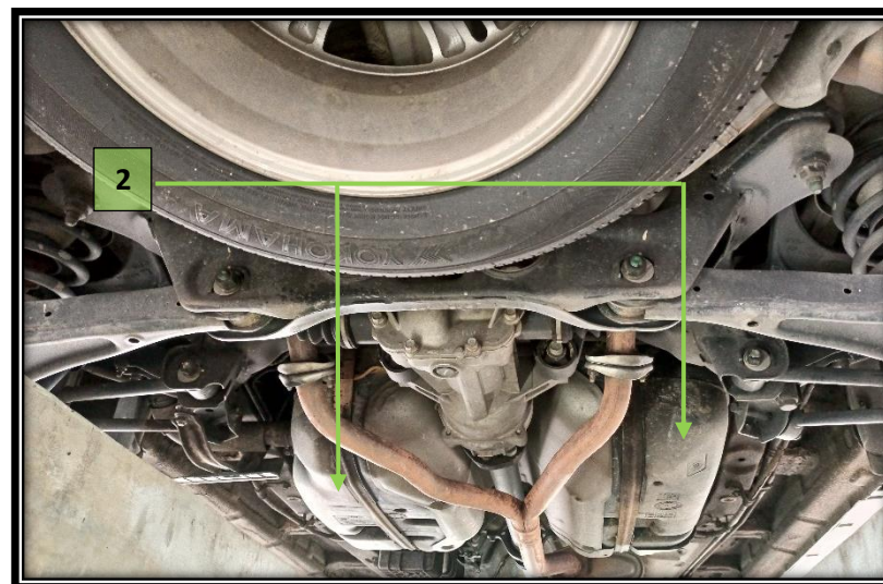
Gambarajah 76 : Komponen Bagi Sistem Bahan Api Inokom Santa-Fe
