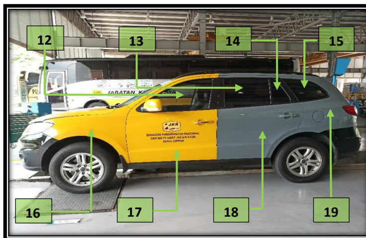
Gambarajah 83 : Komponen Bagi Sistem Badan Kenderaan Inokom Santa-Fe (3)
