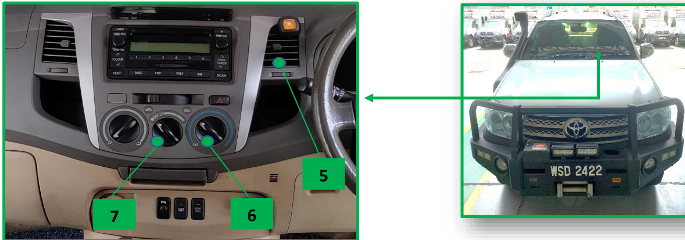
Gambarajah 8 : Komponen Bagi Sistem Penyaman Udara Toyota Fortuner (2)
