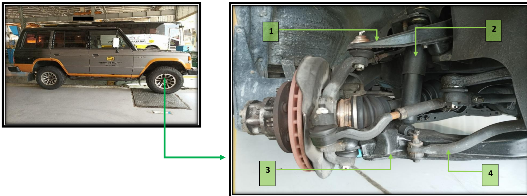
Gambarajah 55 : Komponen Bagi Sistem Suspension Mitsubishi Pajero (1)
