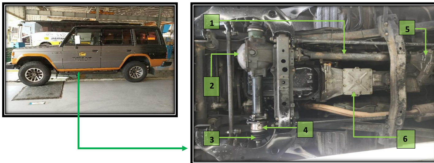
Gambarajah 47 : Komponen Bagi Sistem Tranmisi Mitsubishi Pajero (1)
