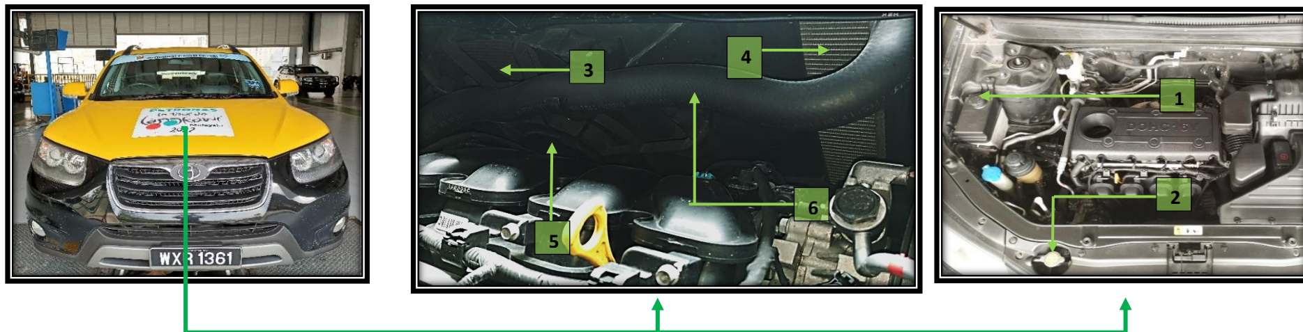
Gambarajah 75 : Komponen Bagi Sistem Penyejukan Inokom Santa-Fe
