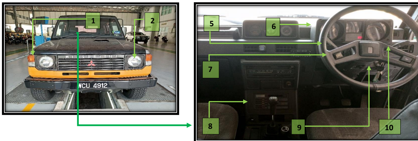
Gambarajah 60 : Komponen Bagi Sistem Elektrikal Mitsubishi Pajero (1)
