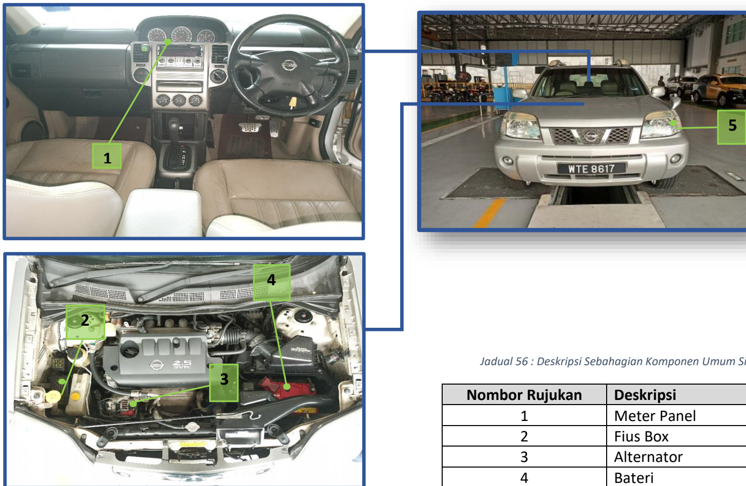
Gambarajah 37 : Komponen Bagi Sistem Elektrikal Nissan Xtrail (1)
