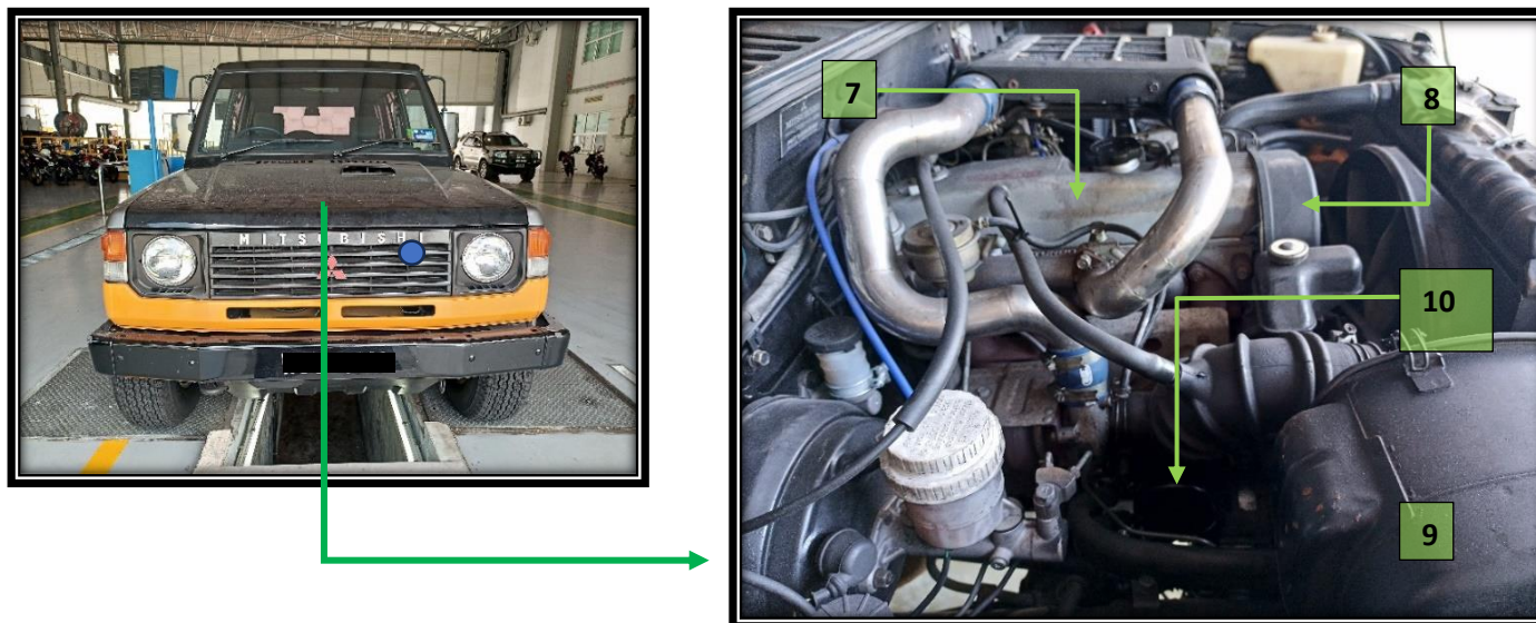
Gambarajah 46 : Komponen Bagi Sistem Enjin Mitsubishi Pajero (2)
