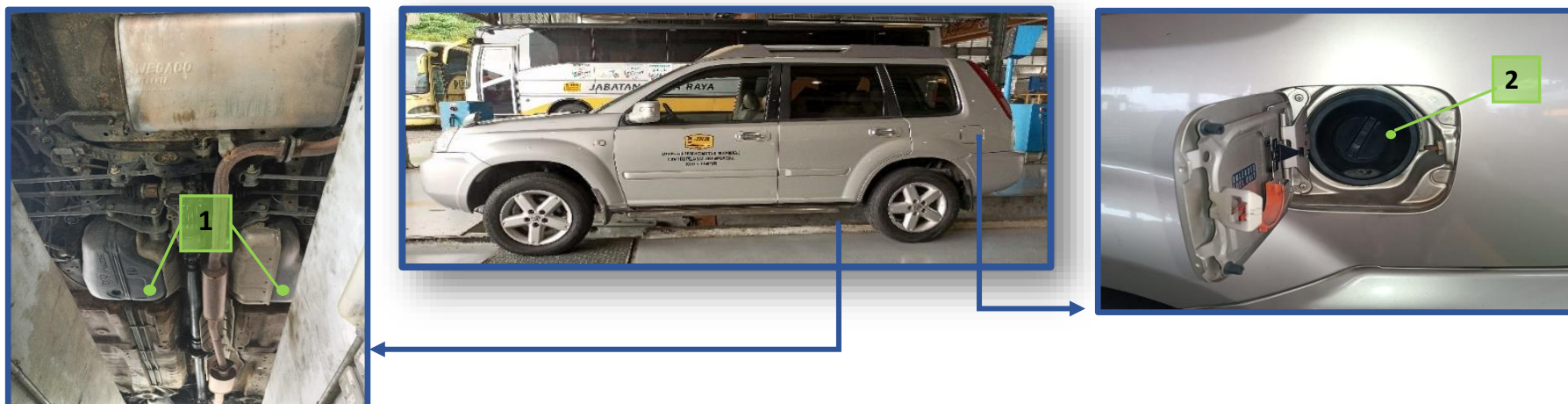
Gambarajah 36 : Komponen Bagi Sistem Bahan Api Nissan Xtrail
