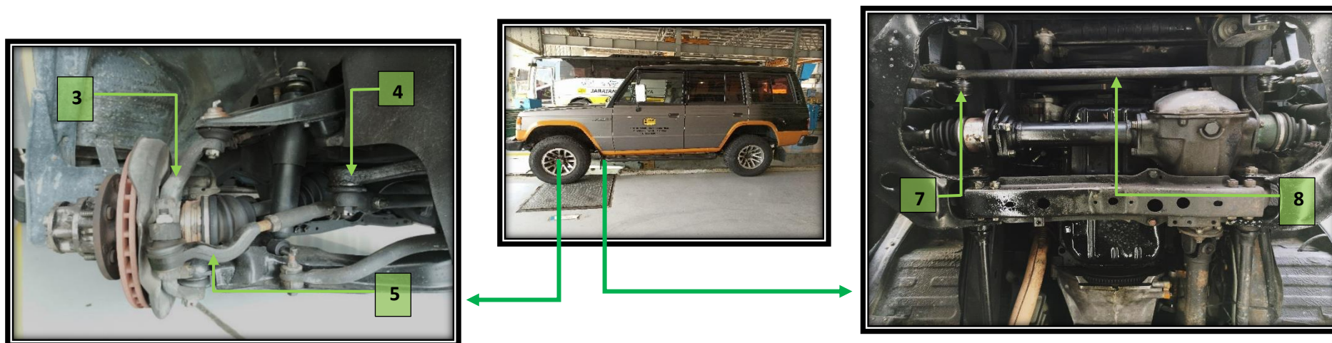
Gambarajah 54 : Komponen Bagi Sistem Stering Mitsubishi Pajero (2)
