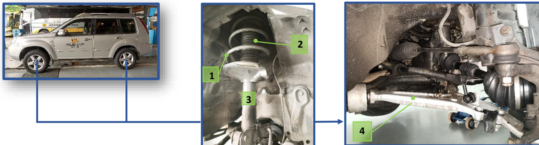
Gambarajah 33 : Komponen Bagi Sistem Suspension Nissan Xtrail (1)
