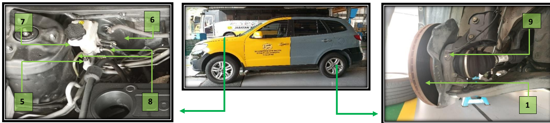
Gambarajah 70 : Komponen Bagi Sistem Brek Inokom Santa-Fe (1)
