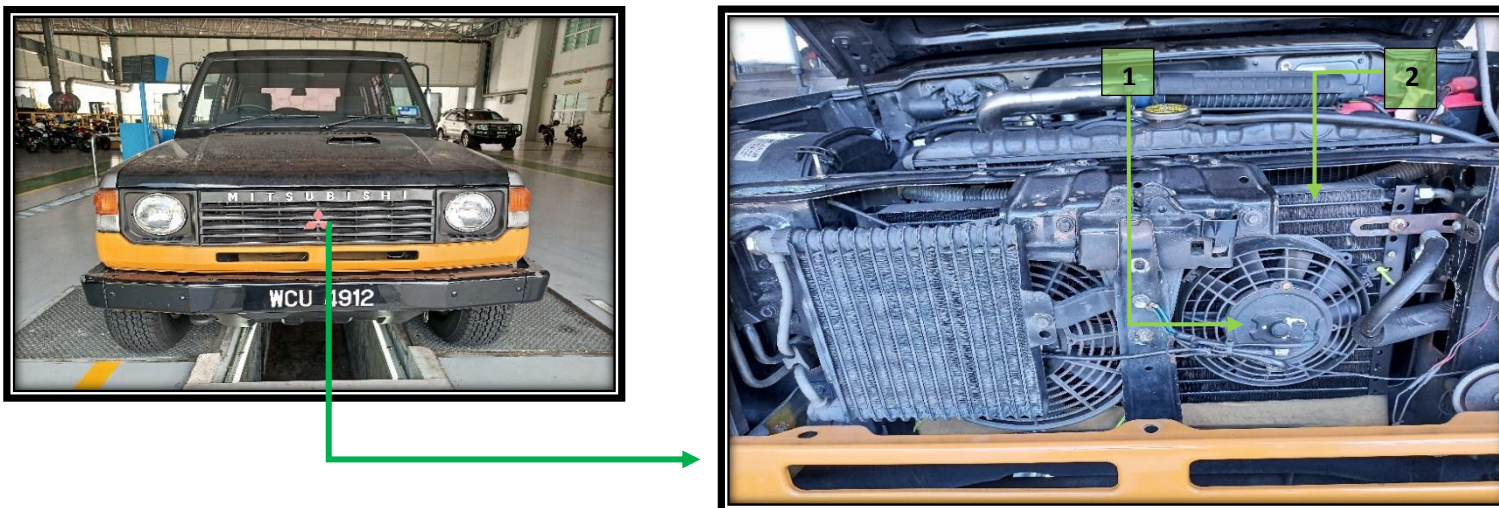
Gambarajah 51 : Komponen Bagi Sistem Penyaman Udara Mitsubishi Pajero (1)
