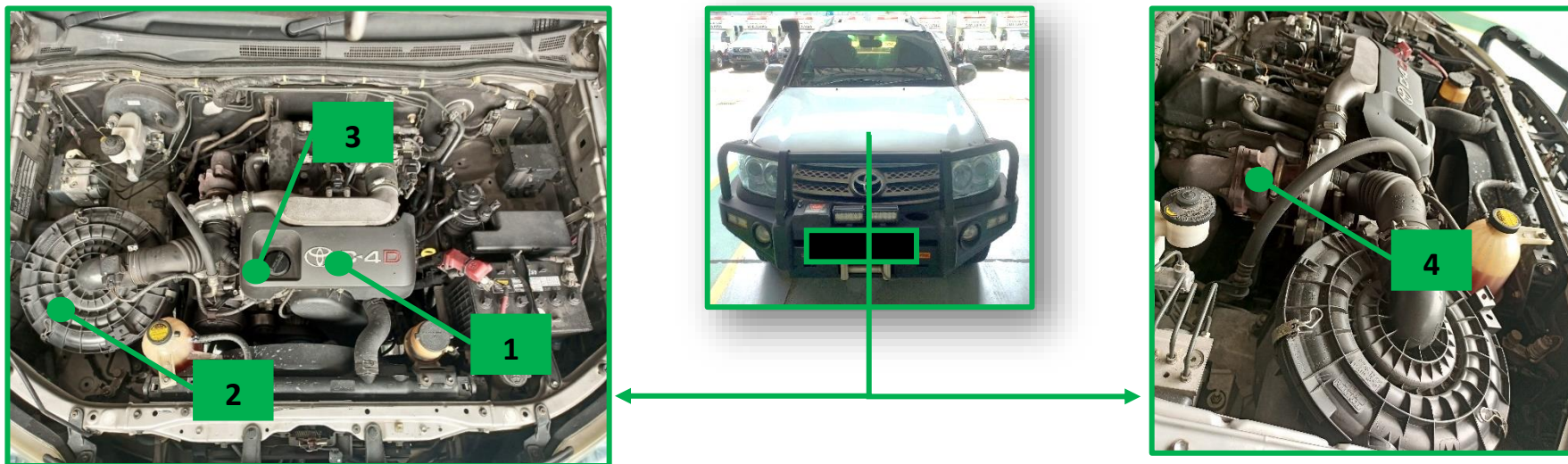
Gambarajah 1 : Komponen Bagi Sistem Enjin Toyota Fortuner (1)
