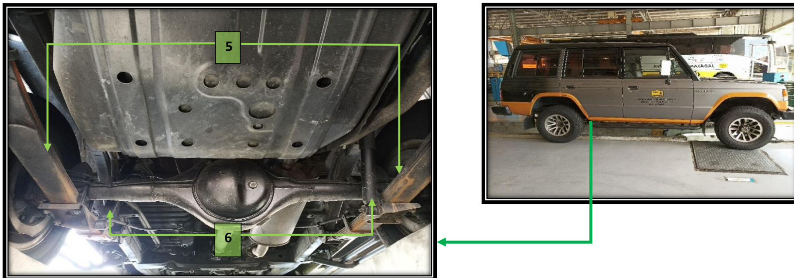
Gambarajah 56 : Komponen Bagi Sistem Suspension Mitsubishi Pajero (2)
