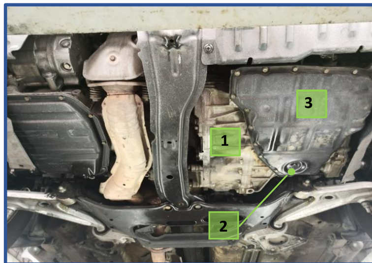
Gambarajah 27 : Komponen Bagi Sistem Tranmisi Nissan Xtrail (1)
