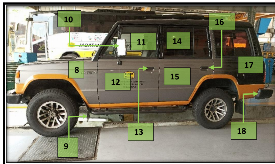
Gambarajah 65 : Komponen Bagi Sistem Badan Kenderaan Mitsubishi Pajero (2)
