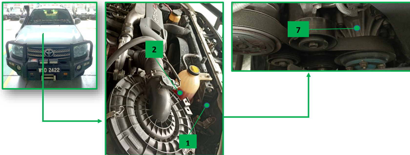
Gambarajah 13 : Komponen Bagi Sistem Penyejukan Enjin Toyota Fortuner (1)
