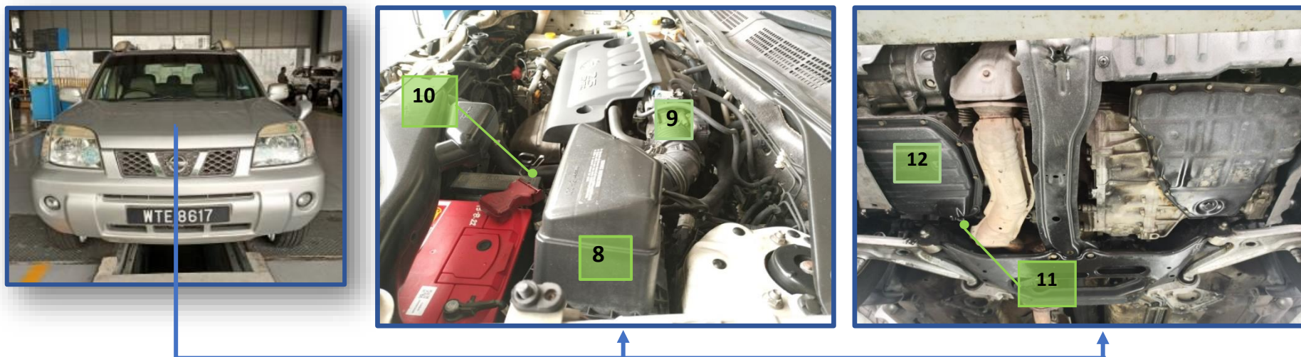
Gambarajah 26 : Komponen Bagi Sistem Enjin Nissan Xtrail (2)
