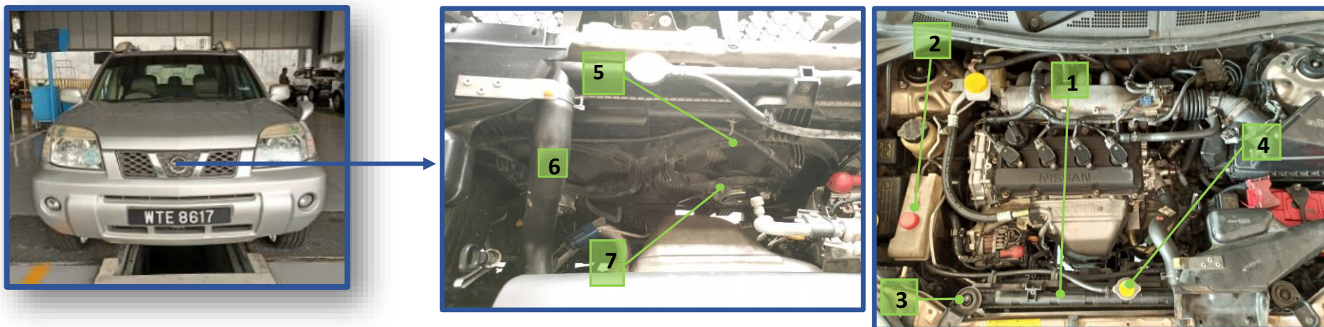
Gambarajah 35 : Komponen Bagi Sistem Penyejukan Nissan Xtrail
