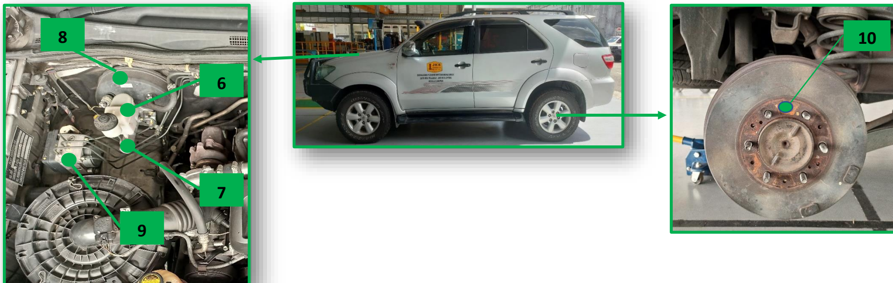
Gambarajah 6 : Komponen Bagi Sistem Brek Toyota Fortuner (2)
