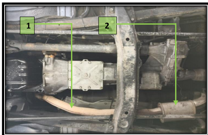
Gambarajah 62 : Komponen Bagi Sistem Ekzos Mitsubishi Pajero
