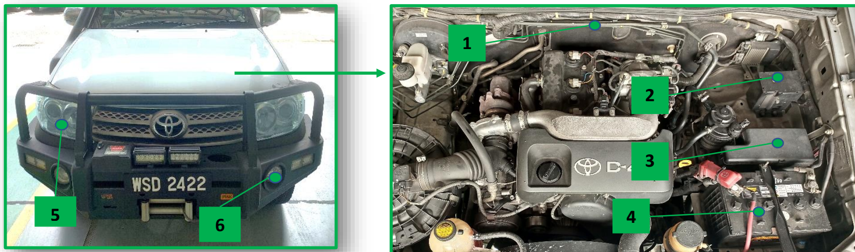
Gambarajah 16 : Komponen Bagi Sistem Elektrikal Toyota Fortuner (1)
